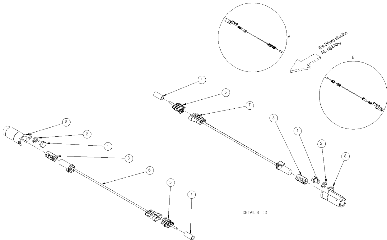
DETAIL A 1:3
